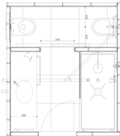
Cellula Bagno con doccia
