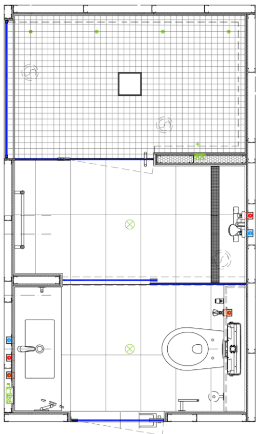
Cellula Bagno con doccia e sauna
