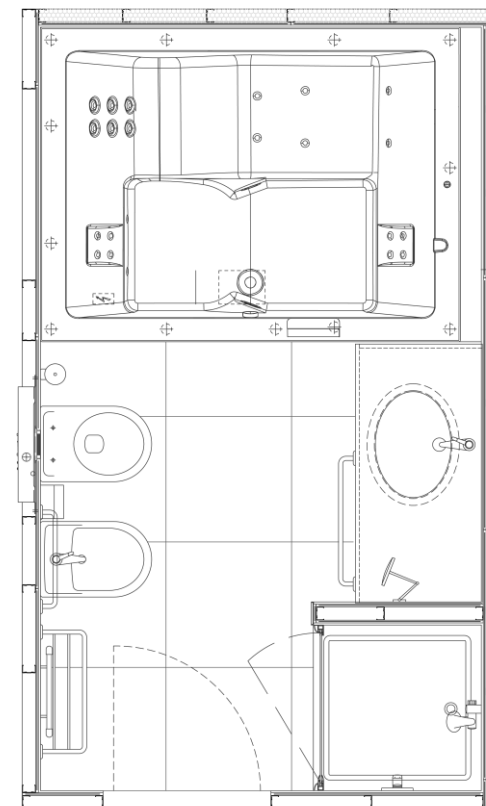
Cellula Bagno con vasca idromassaggio doppia, doccia e tv integrata
